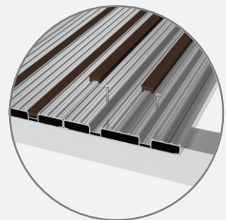
볼트커버 시공 (피스 매립형 체결)
