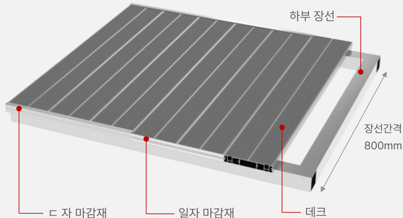
(혁신제품) 데크 + 데크커버(플랫형)
