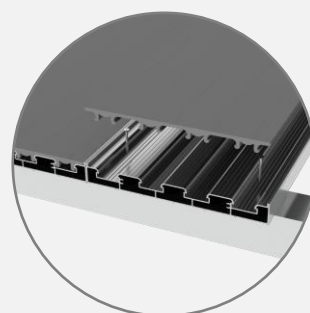
데크 + 데크커버(플랫형) (피스 매립형 체결)
