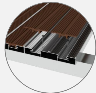
데크 + 데크커버(논슬립형) (피스 매립형 체결)
