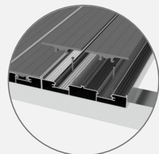
데크 + 데크커버(플랫형) (피스 매립형 체결)
